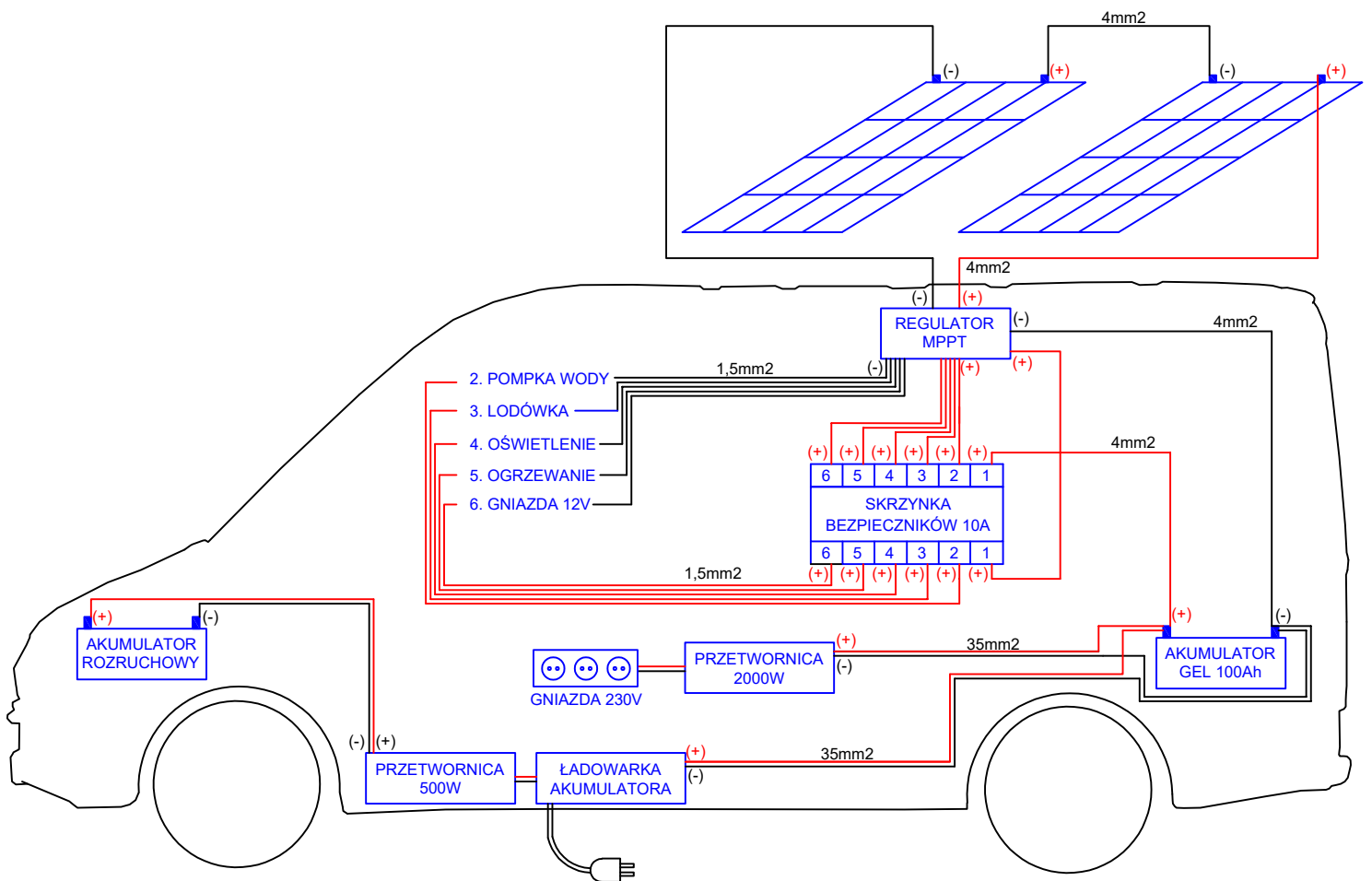
SCHEMAT INSTALACJI ELEKTRYCZNEJ VANDALVAN.COM
